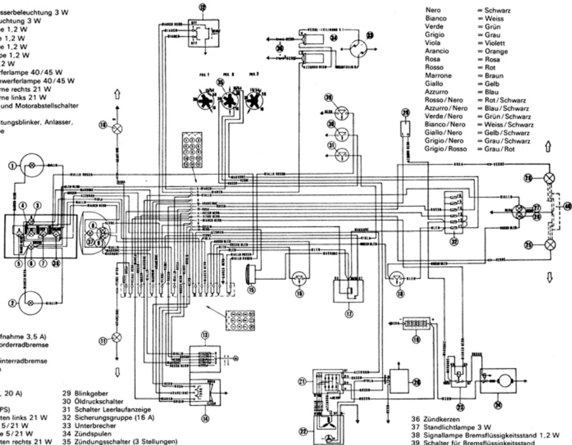
Bild 395 Schaltplan Modell 850 Le Mans
