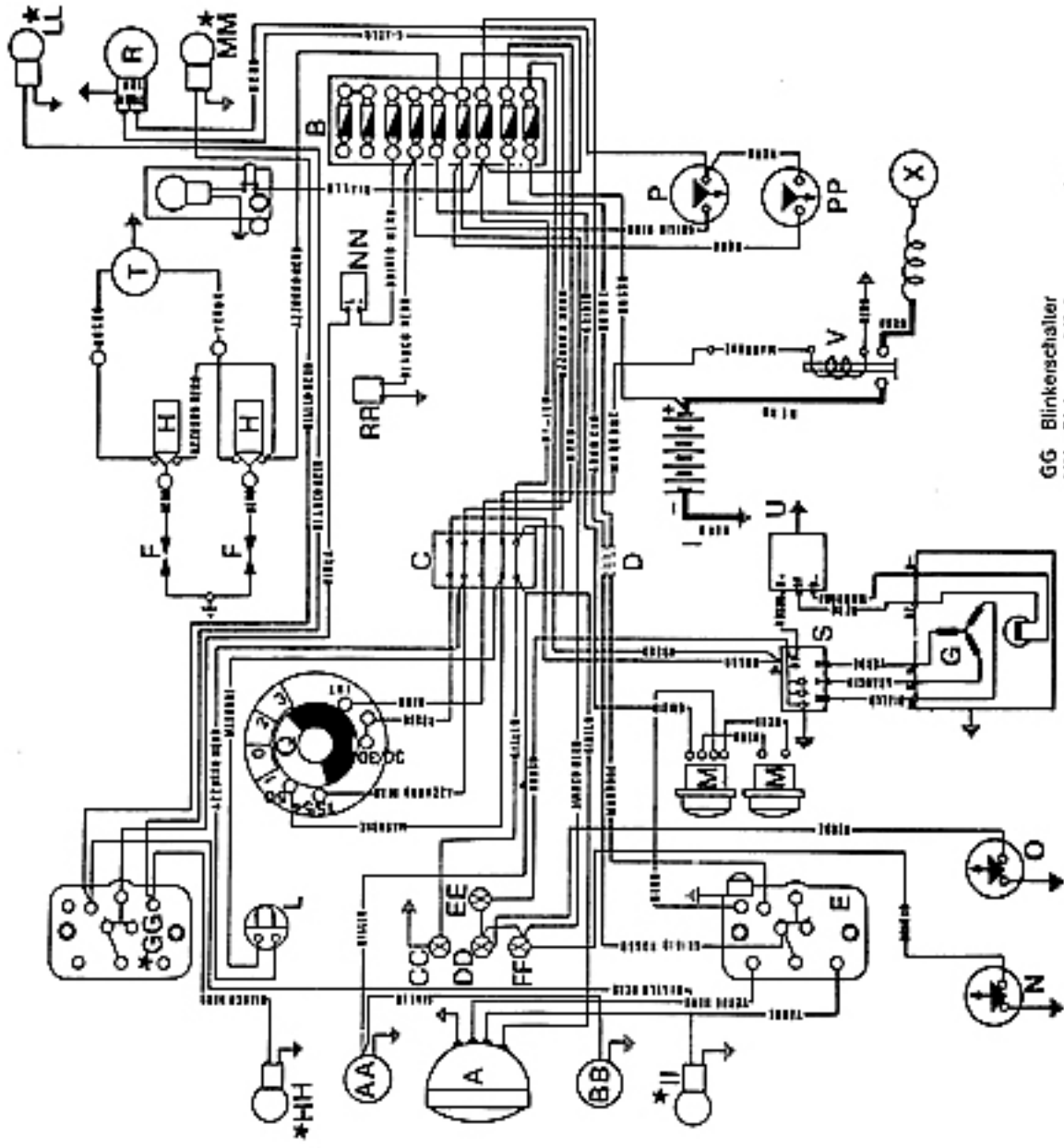
Bild 391 Schaltplan Modell 750-S
